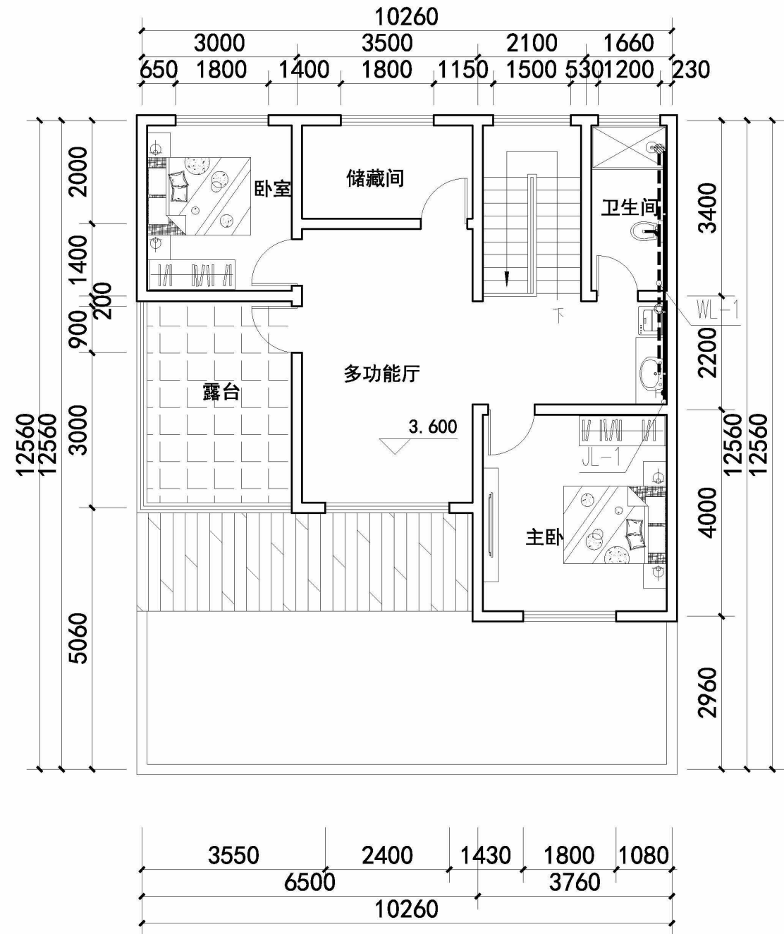
二层平面图 1:100
