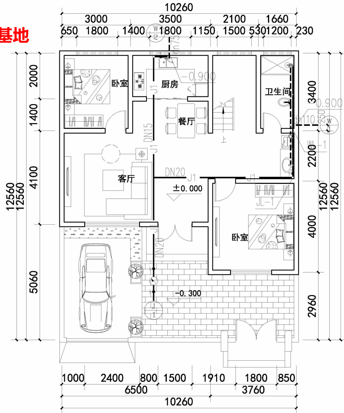
一层平面图 1:100
